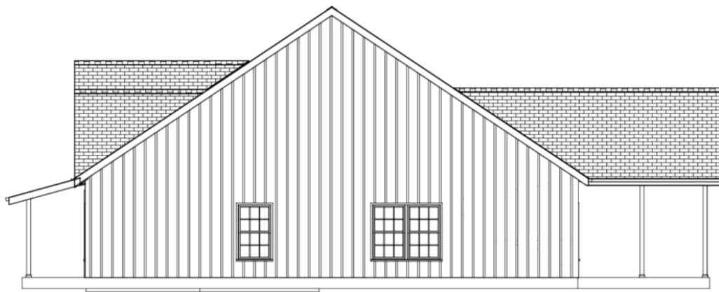
Elevation 3
